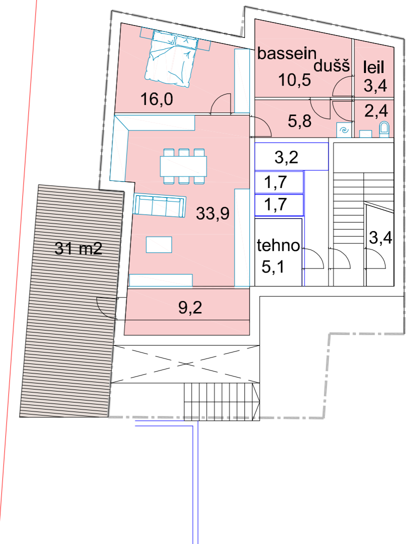
-1. korrus - 82 m 2
